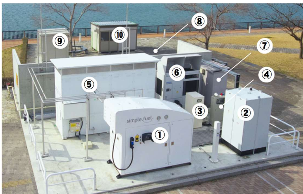
図4 “水素ステーションおおい うみんぴあ”の設備（①～⑩の設備名称は、本文中のものに対応）
